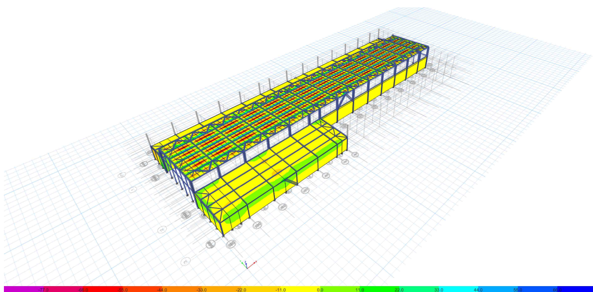
Eforturi principale S22
