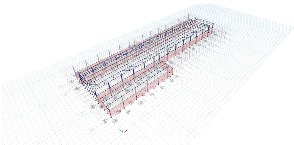
Forte taietoare V3 - infasuratoare
