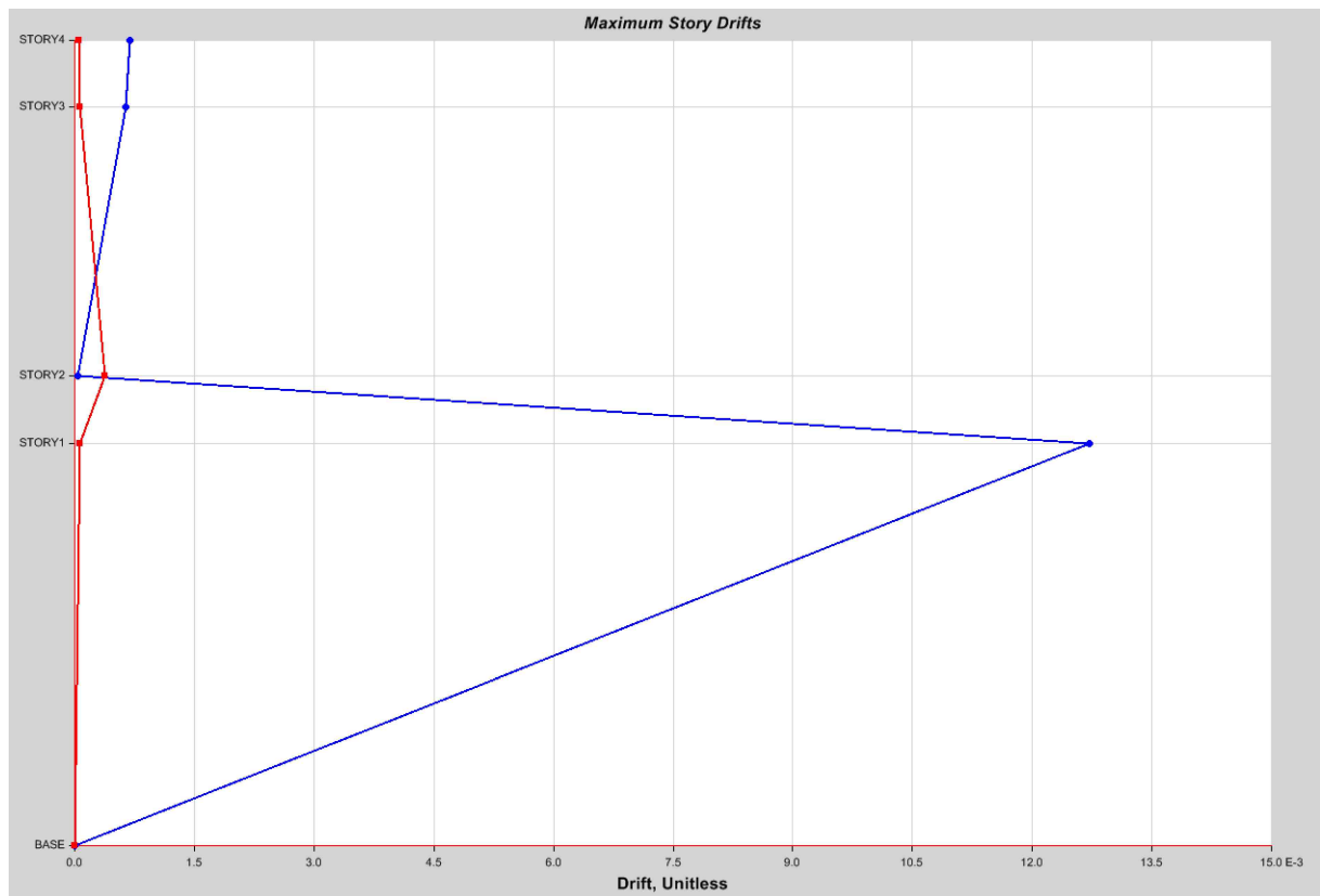
Rotiri relative de nivel seism x
