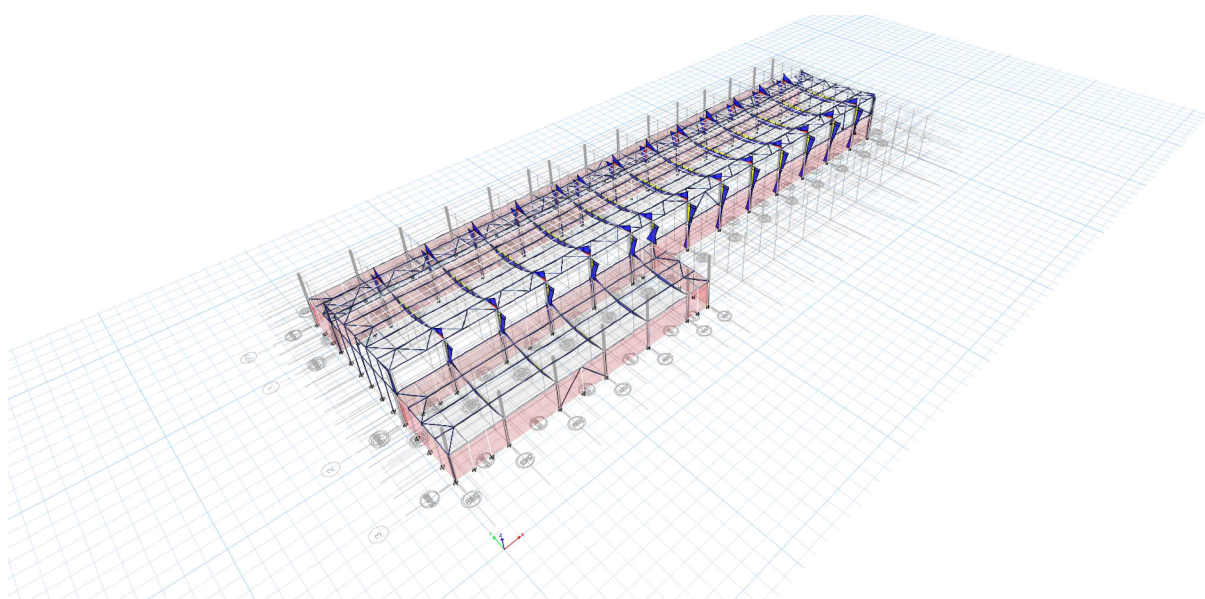
Momente incovoietoare M3 - infasuratoare
