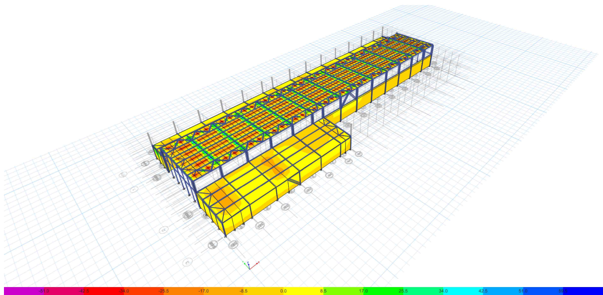
Eforturi principale S11
