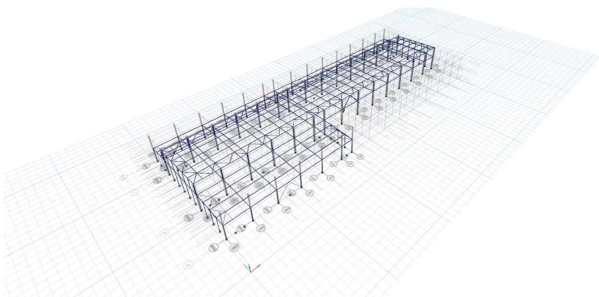
Forte taietoare V3 - infasuratoare
