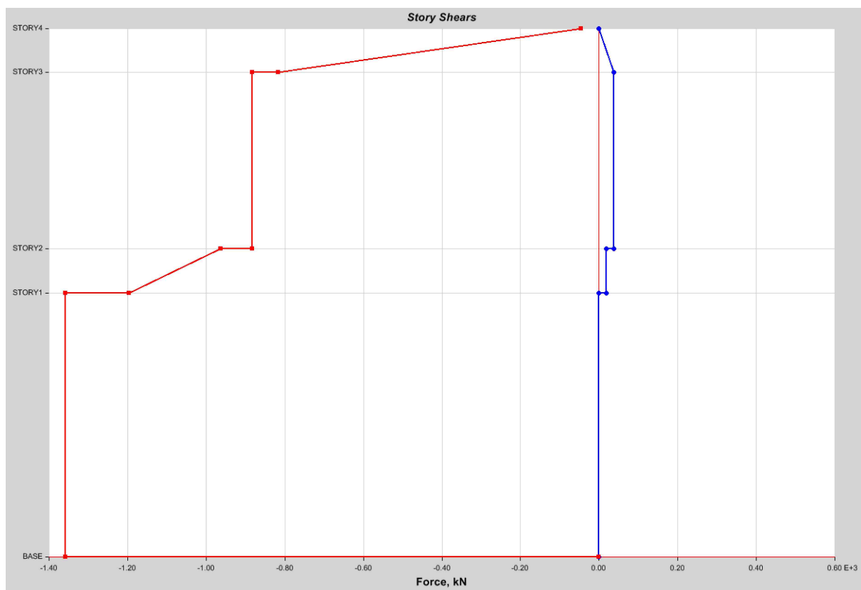
Fora taietoare seism y
