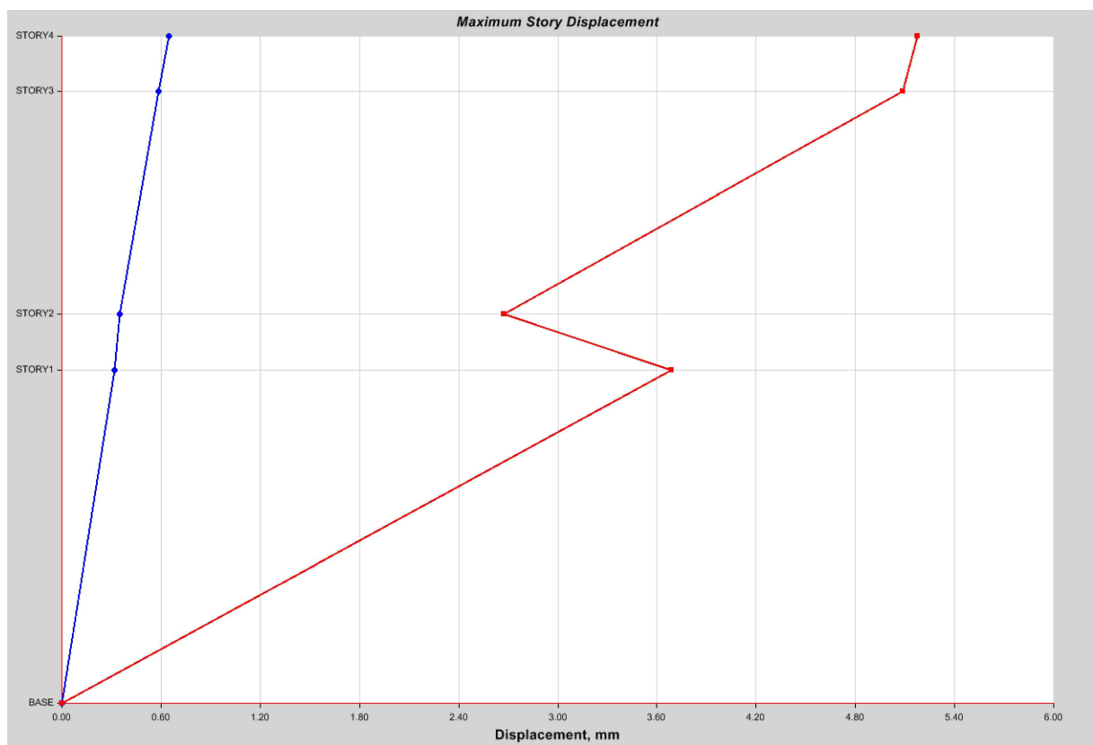
Deformatii absolute seism y
