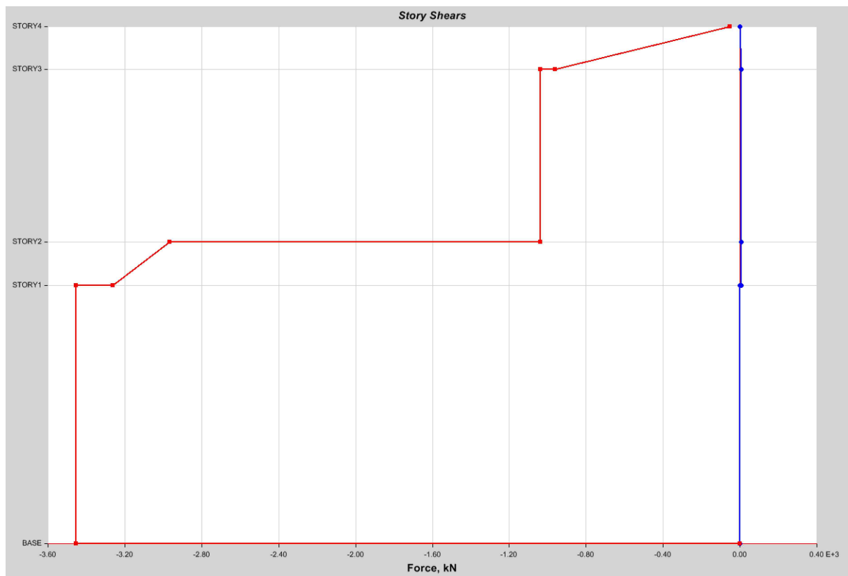
Fora taietoare seism y
