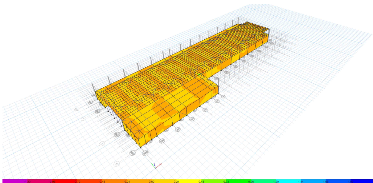
Eforturi principale S13
