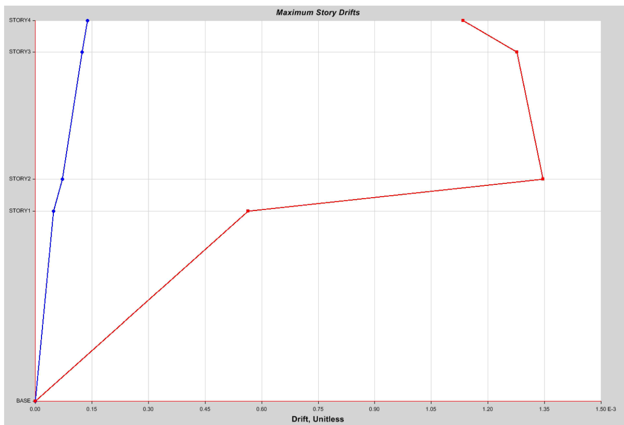
Rotiri relative de nivel seism y
