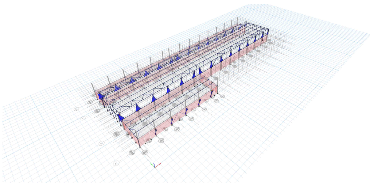
Momente incovoietoare M2 - infasuratoare
