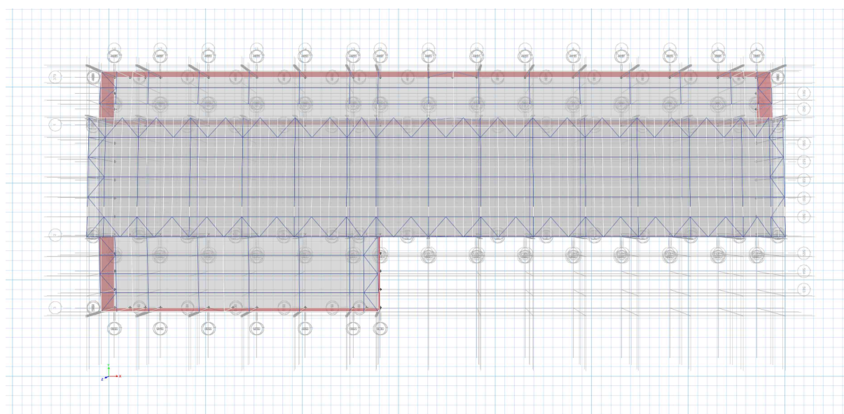
Model de calcul structural – vedere 2
