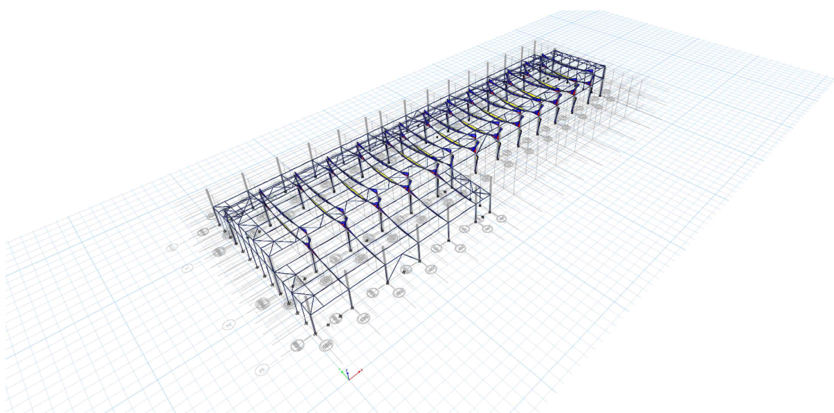
Momente incovoietoare M3 - infasuratoare
