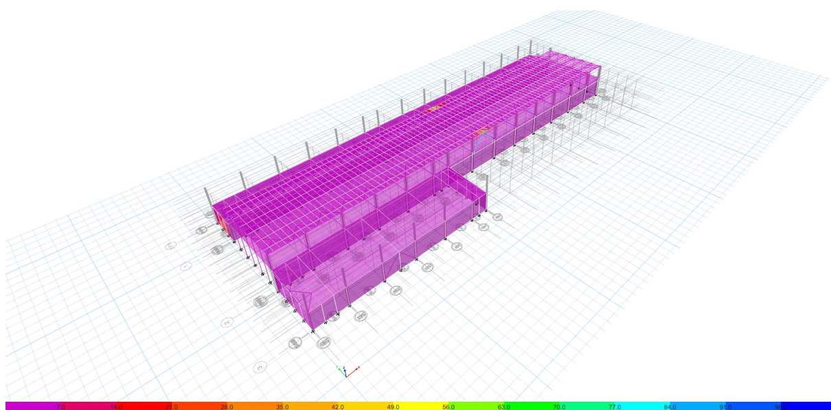
Energie disipata seism x
