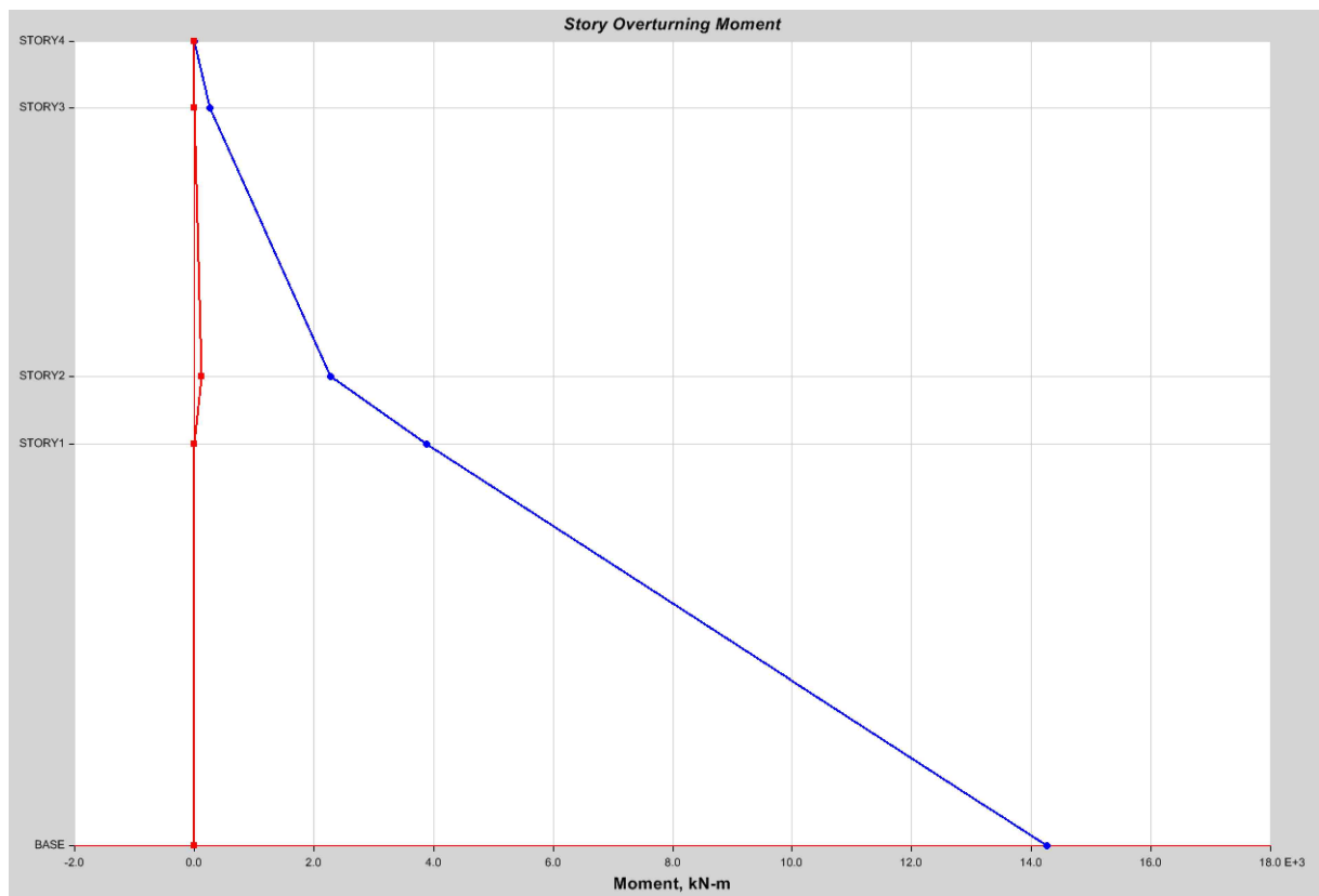
Moment de rasturnare seism y
